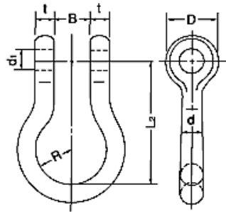
■RBシャックルの本体
